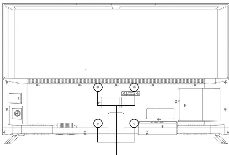
掛け金具取付用ネジ穴 (200mm×200mm)
