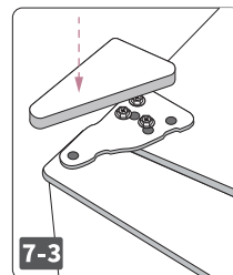
ヒンジカバーを上から被せて取り付けます。
