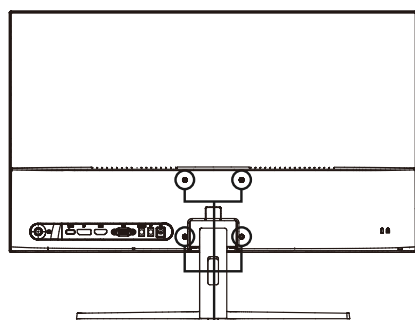
壁掛け金具取付用ネジ穴
