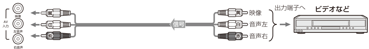
接続例
